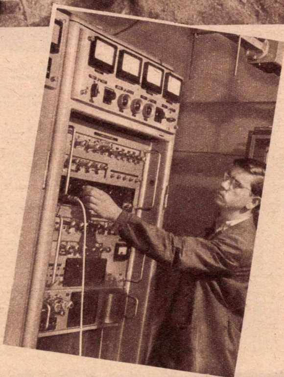
Részlet a kékesi adóberendezésből (Egri Gyula felvétele)
